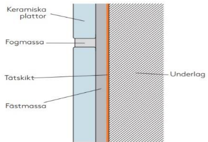
Figur 2. Principskiss vägg.
