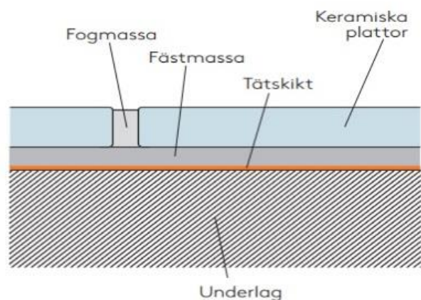
Figur 1. Principskiss golv.
