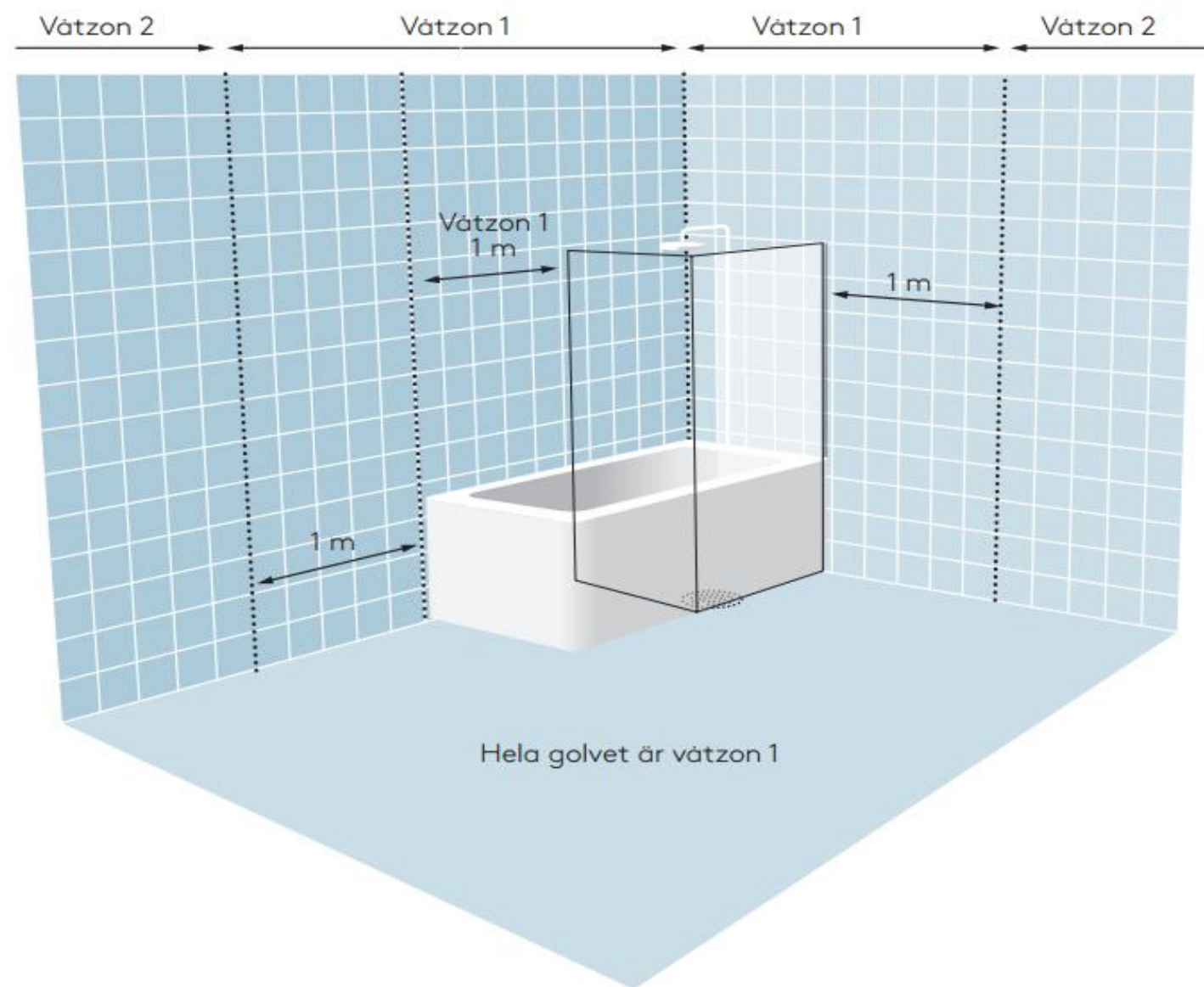
Figur 5. Våtzoneindelning våtrum.
